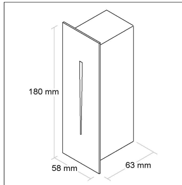
DIMENSÃO - BL6007
