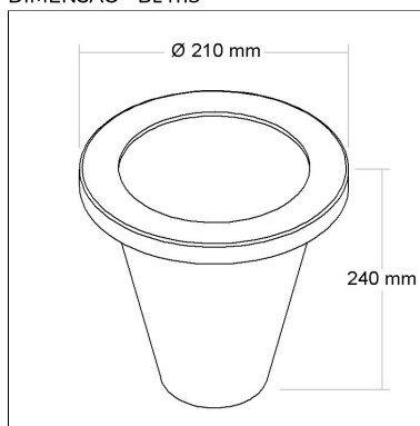
DIMENSÃO - BL4113
