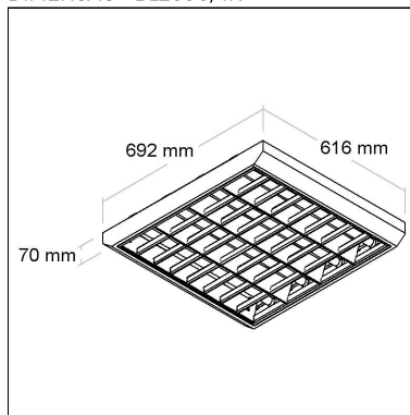
DIMENSÃO - BL2090/4K
