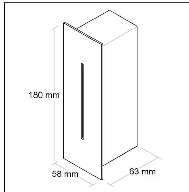
DIMENSÃO - BL6006
