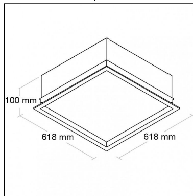
DIMENSÃO - BL1274/3K
