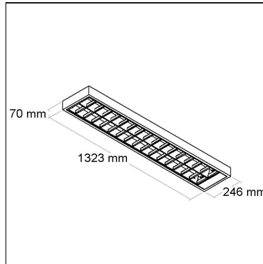
DIMENSÃO - BL2091/G5
