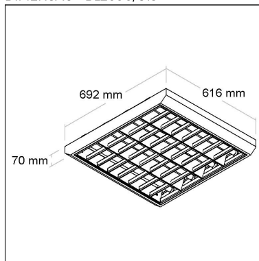
DIMENSÃO - BL2090/G13
