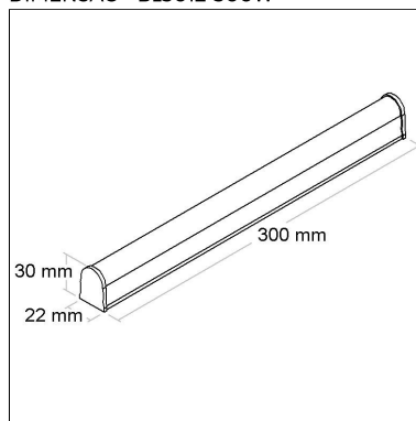
DIMENSÃO - BL3012-300W
