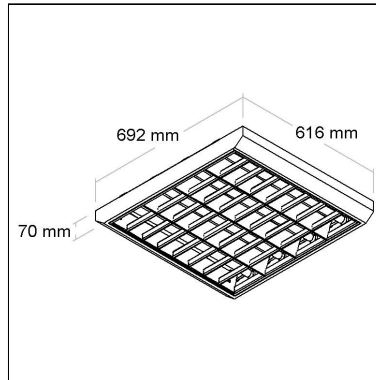
DIMENSÃO - BL2090/G5
