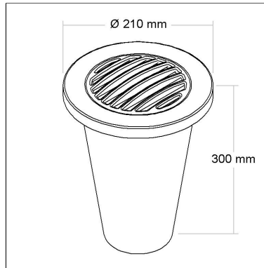
DIMENSÃO - BL4117G
