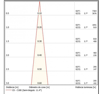
ILUMINÂNCIA - BL1581
