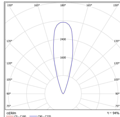
FOTOMETRIA - BL4109/208W
