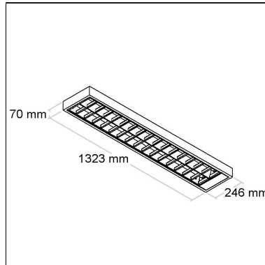
DIMENSÃO - BL2091/G13
