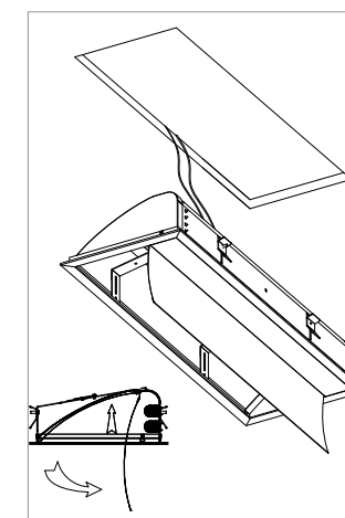
Refletor basculante que permite o acesso a área interna da luminária
