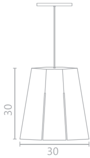
Ref. 109 D - 30 cm A - 30 cm 1X E-27 Económica 25W
