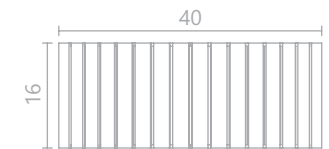
Ref. 4039 L - 40 cm A - 16 cm P - 10 cm 2X E-27 Económica 25W
