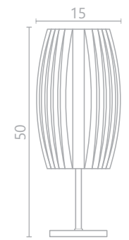
Ref. 7011 D - 15 cm A - 50 cm 1X E-27 Económica 25W
