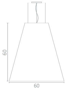
Ref. 1154 D - 60 cm A - 60 cm 4X E-27 Económica 25W
