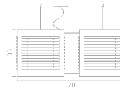
Ref. 120 L - 70 cm A - 30 cm P - 30 cm 2X E-27 Económica 25W
