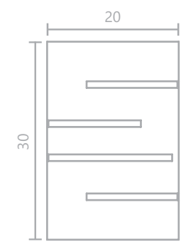
Ref. 4060 L - 20 cm A - 30 cm P - 8,5 cm 2X E-27 Económica 25W
