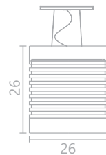
Ref. 800 L - 26 cm A - 26 cm P - 26 cm 1X E-27 Econômica 25W
