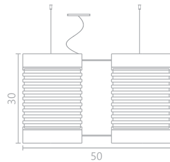
Ref. 804 L - 50 cm A - 30 cm P - 19 cm 2X E-27 Econômica 25W
