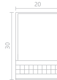
Ref. 443 L - 20 cm A - 30 cm P - 9,5 cm 1X E-27 Económica 25W
