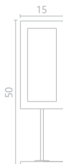
Ref. 616 L - 15 cm A - 50 cm P - 15 cm 1X E-27 Económica 25W
