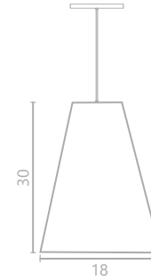
Ref. 1214 D - 18 cm A - 30 cm 1X E-27 Económica 25W
