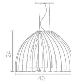
Ref. 1187 D - 40 cm A - 24 cm 1X E-27 Económica 25W
