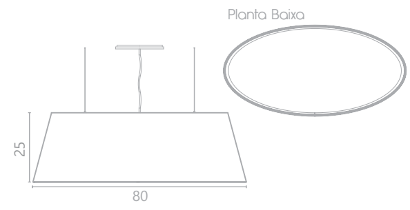
Ref. 1218A L - 80 cm A - 25 cm P - 40 cm 6X E-27 Económica 25W
