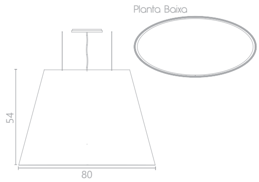
Ref. 1219A L - 80 cm A - 54 cm P - 40 cm 6X E-27 Económica 25W
