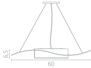
Ref. 1108 L - 60 cm A - 6,5 cm P - 35 cm 2X E-27 Económica 25W
