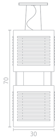
Ref. 110 L - 30 cm A - 70 cm P - 30 cm 2X E-27 Económica 25W
