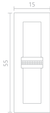
Ref. 439 L - 15 cm A - 55 cm P - 9,5 cm 2X E-27 Económica 25W
