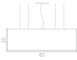
Ref. 287 L - 82 cm A - 25 cm P - 45 cm 6X E-27 Económica 25W
